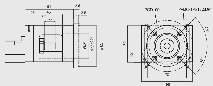
Moduł KK100 Kołnierz łączący F5
