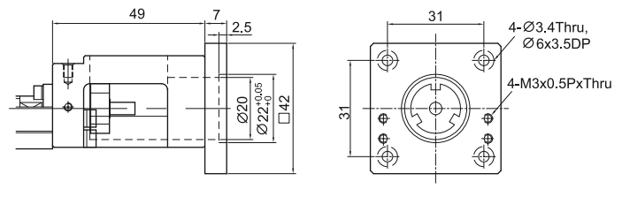
Moduł KK40 Kołnierz łączący F3
