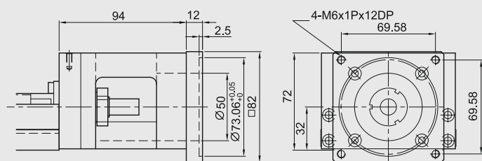
Moduł KK100 Kołnierz łączący F4
