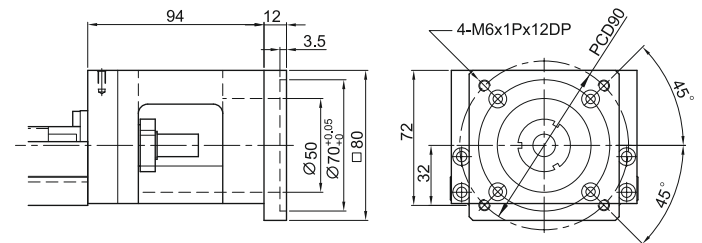
Moduł KK100 Kołnierz łączący F1
