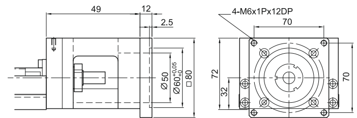
Moduł KK100 Kołnierz łączący F3
