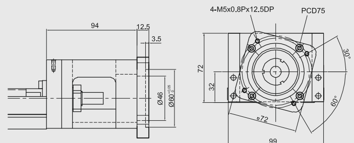
Moduł KK100 Kołnierz łączący F7
